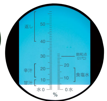
そば・うどん用濃度計目盛
